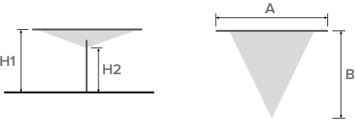
STRUCTURE TRIANGULAIRE
